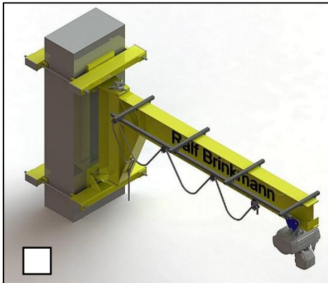
Mit Stützenumfassungskonsolle
