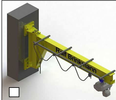
Mit Wandkonsolenplatten
